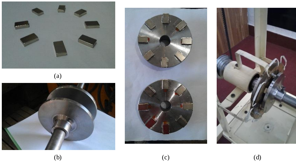
Figure 7. Neodymium permanent magnets (b) Rotor plates (c) Rotor discs (d) Complete AFPMG model.
